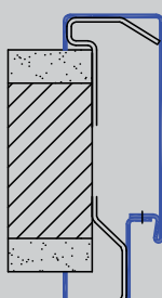
2-részes tok minden faltípushoz
