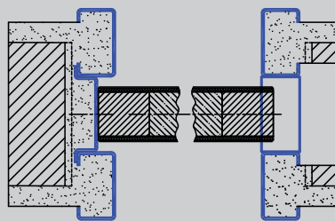
Falban futó tolótok (vízszintes metszet)
