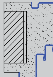
Dupla falcos átfogótok egy oldali vakoló horonnyal
