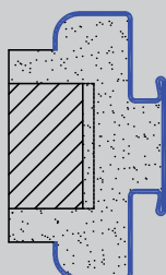
Rádiuszos átfogótok két ajtólapozhoz
