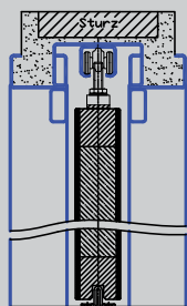
Falban futó tolótok (függőleges metszet)
