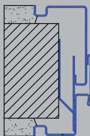
2-részes tok állítható falvastag- sággal és vakolóhorronnyal
