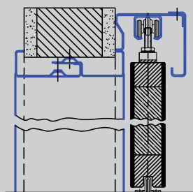
Fal előtt futó tolótok 2-részes kivitel
