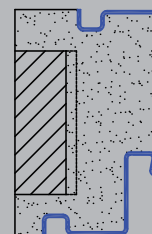
Átfogótok vakoló horonnyal
