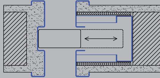
Tolótok készdoboz rendszerhez
