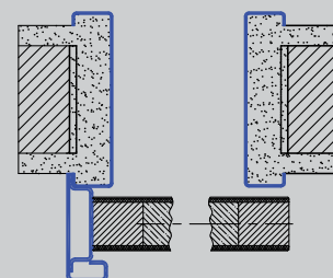
Fal előtt futó tolótok (vízszintes metszet)
