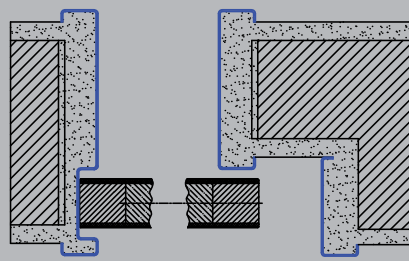
Falnyílásban futó tolótok
