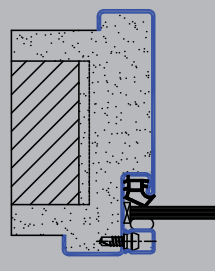
Ablakkeret 1-oldali üvegezéshez
