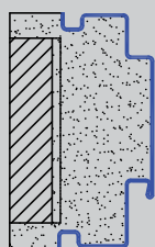
Díszfalcos átfogótok vakoló horonnyal
