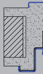
Ólombetétes tok
