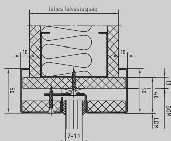
1-es típus
