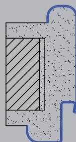
Rádiuszos átfogótok
