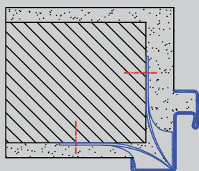
Saroktok rögzítése
