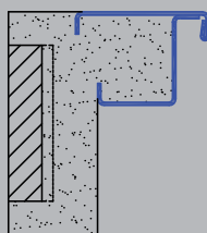
Tornacsarok saroktok
