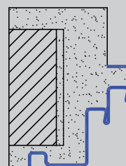
Dupla falcos saroktok vakoló horonnyal
