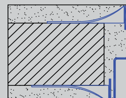
Toktükrő nélküli tok
