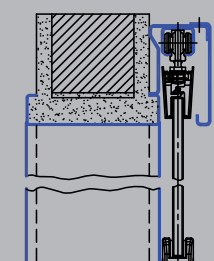
Fal előtt futó tolótok üveg ajtóval
