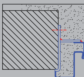
Saroktok beépítése
