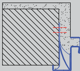
Saroktok rögzítése
