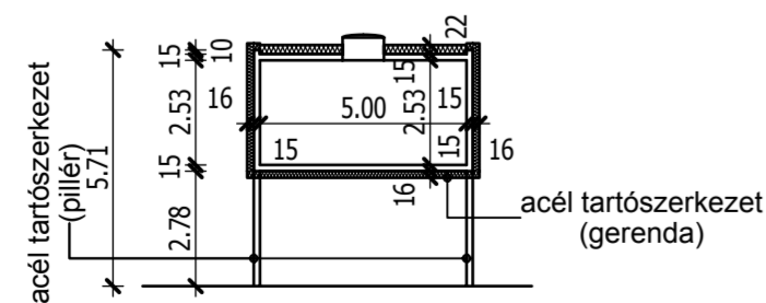
ÖSSZEKÖTŐ FOLYOSÓ METSZET M=1:200
