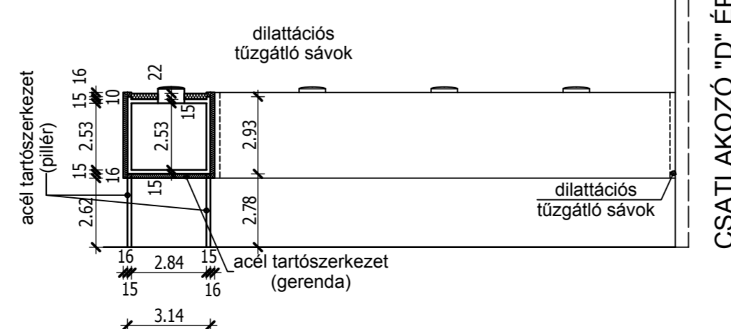
ÖSSZEKÖTŐ FOLYOSÓ METSZET ÉS HOMLOKZAT M=1:200
